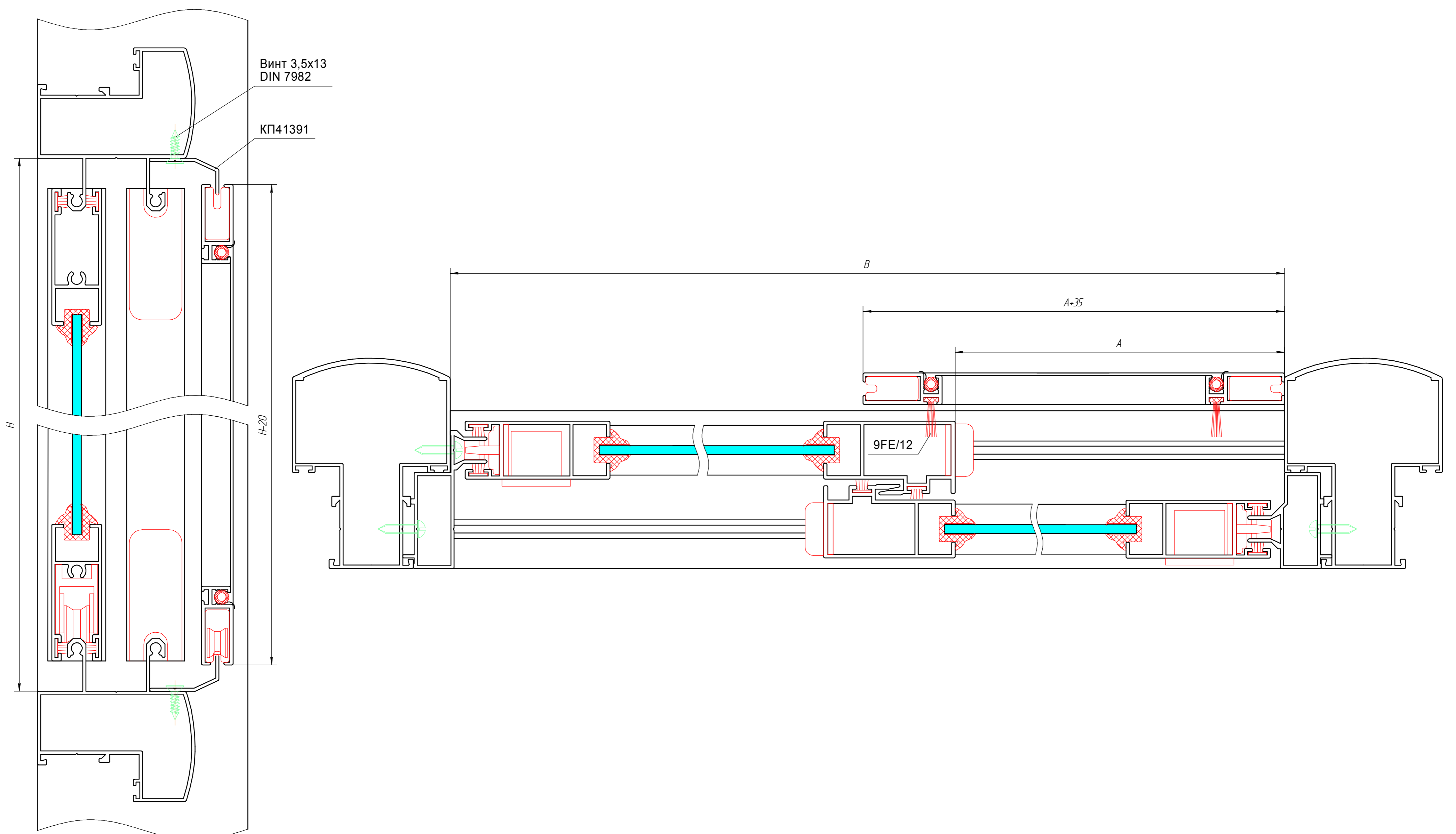
Монтаж раздвижной москитной сетки в систему КП47 с наружным пилоном.
