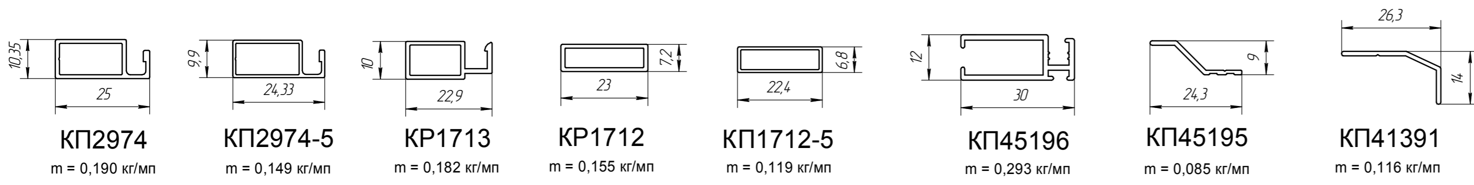
Монтаж москитной сетки в систему КП47
